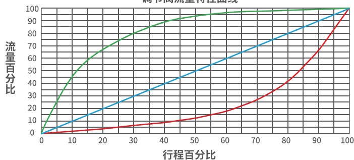
调节阀流量特性曲线
