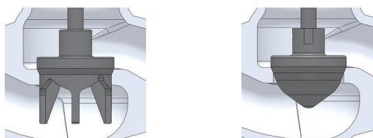
I V口阀芯, 精准控制流量。 II 抛物线型阀芯, 快速调节流量。
